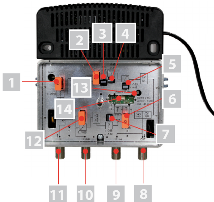
Bild 2: Verstärker HV 12E3625, Innenansicht (andere Typen ähnlich)
