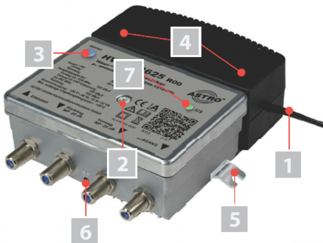
Bild 1: Verstärker HV 12E3625 (andere Typen ähnlich)
